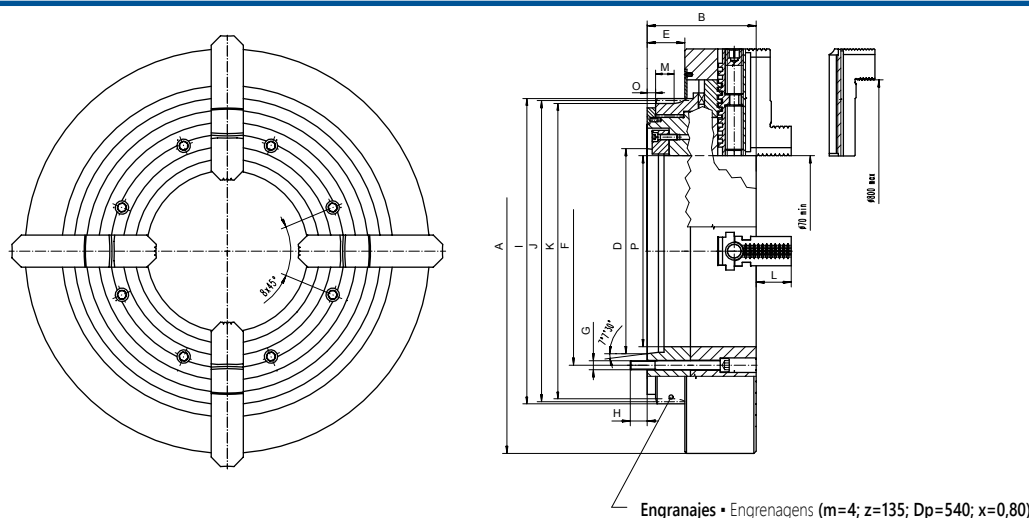
Engranajes • Engrenagens (m=4; z=135; Dp=540; x=0,80)
