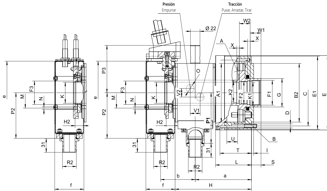
SDC - Estándar con control de carrera de pistón mediante dos interruptores de proximidad
