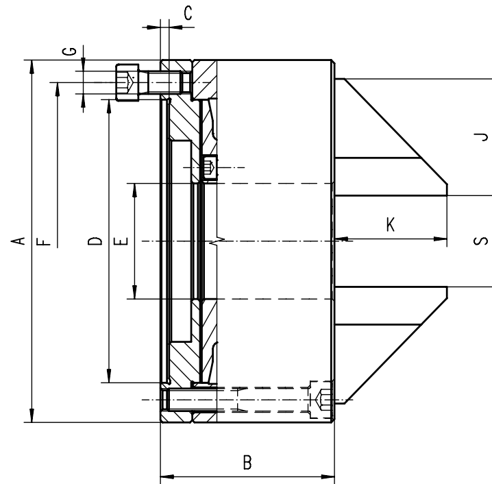
Plato 160mm Tamanho do mandril 160mm
